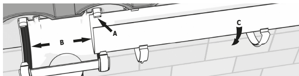
Рис. 3: Установка водосточного желоба
